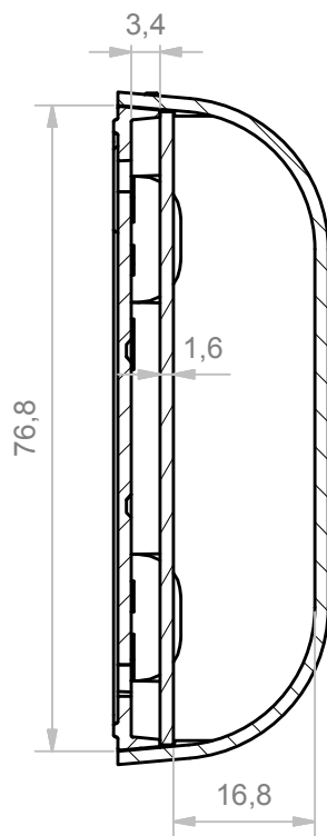
A-A (1:1)
